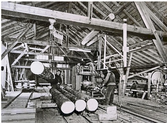
Der Gatterbetrieb im Schwalefelder Sägewerk. Rundholz wird aufgeschnitten.
